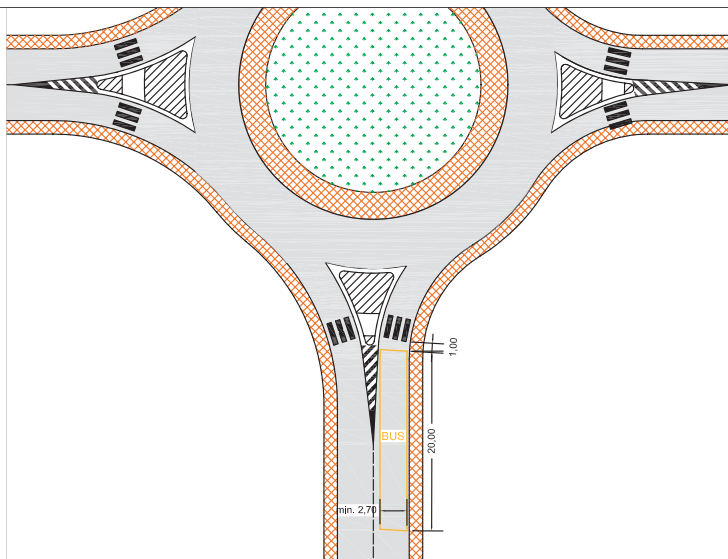
Schema raccomandato per l'organizzazione delle fermate del Trasporto Pubblico Locale su gomma per classe funzionale stradale
