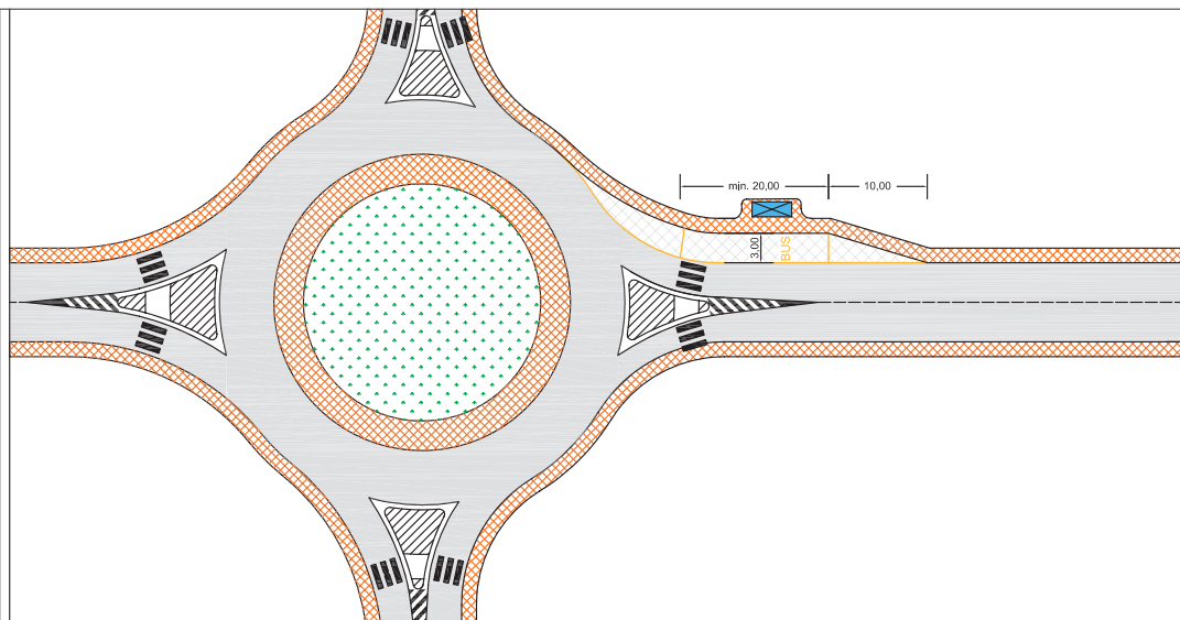
Schema raccomandato per l'organizzazione delle fermate del Trasporto Pubblico Locale su gomma per classe funzionale stradale
